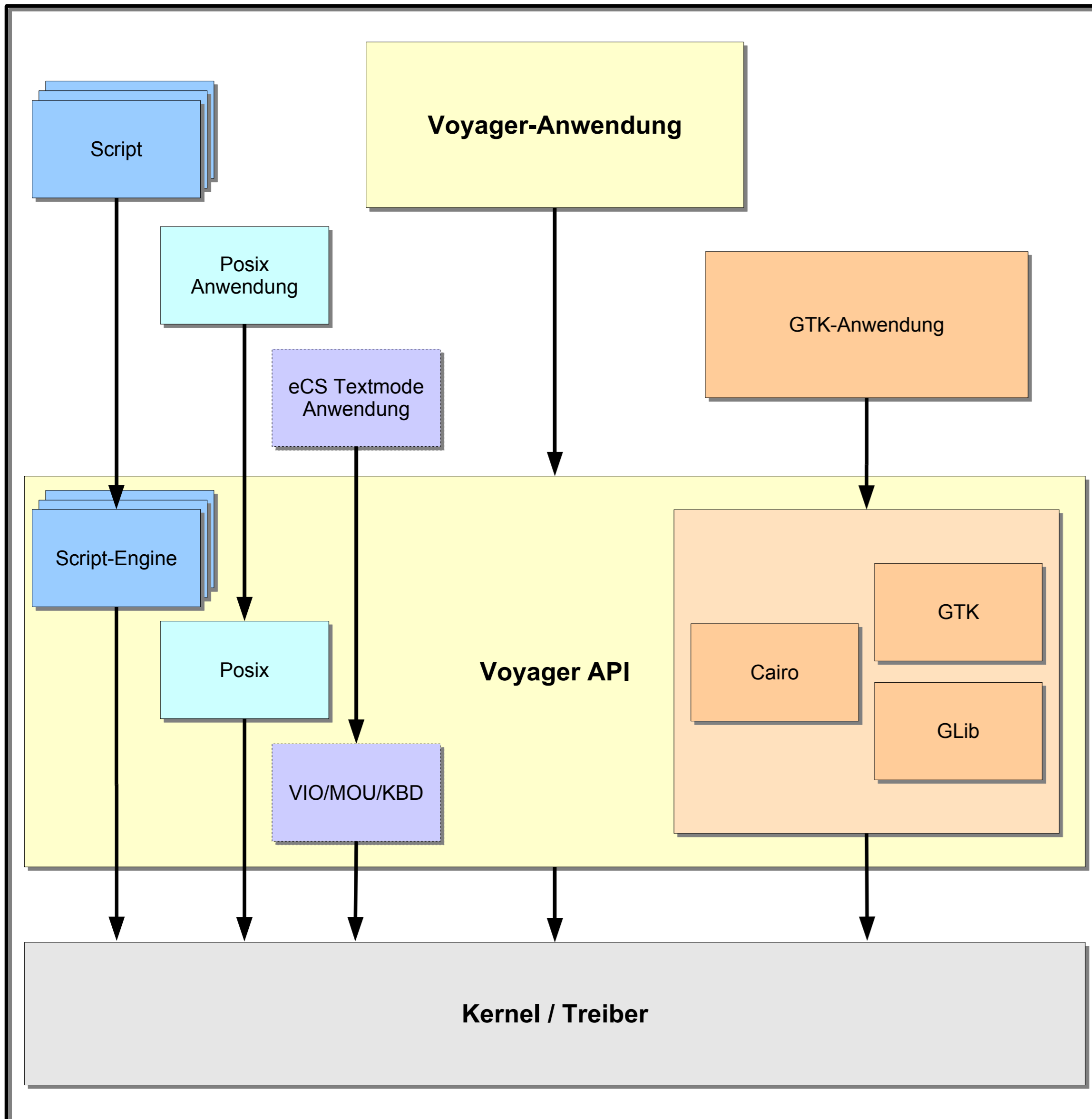
Voyager API: Mögliche Variante des Zusammenspiels der Komponenten
