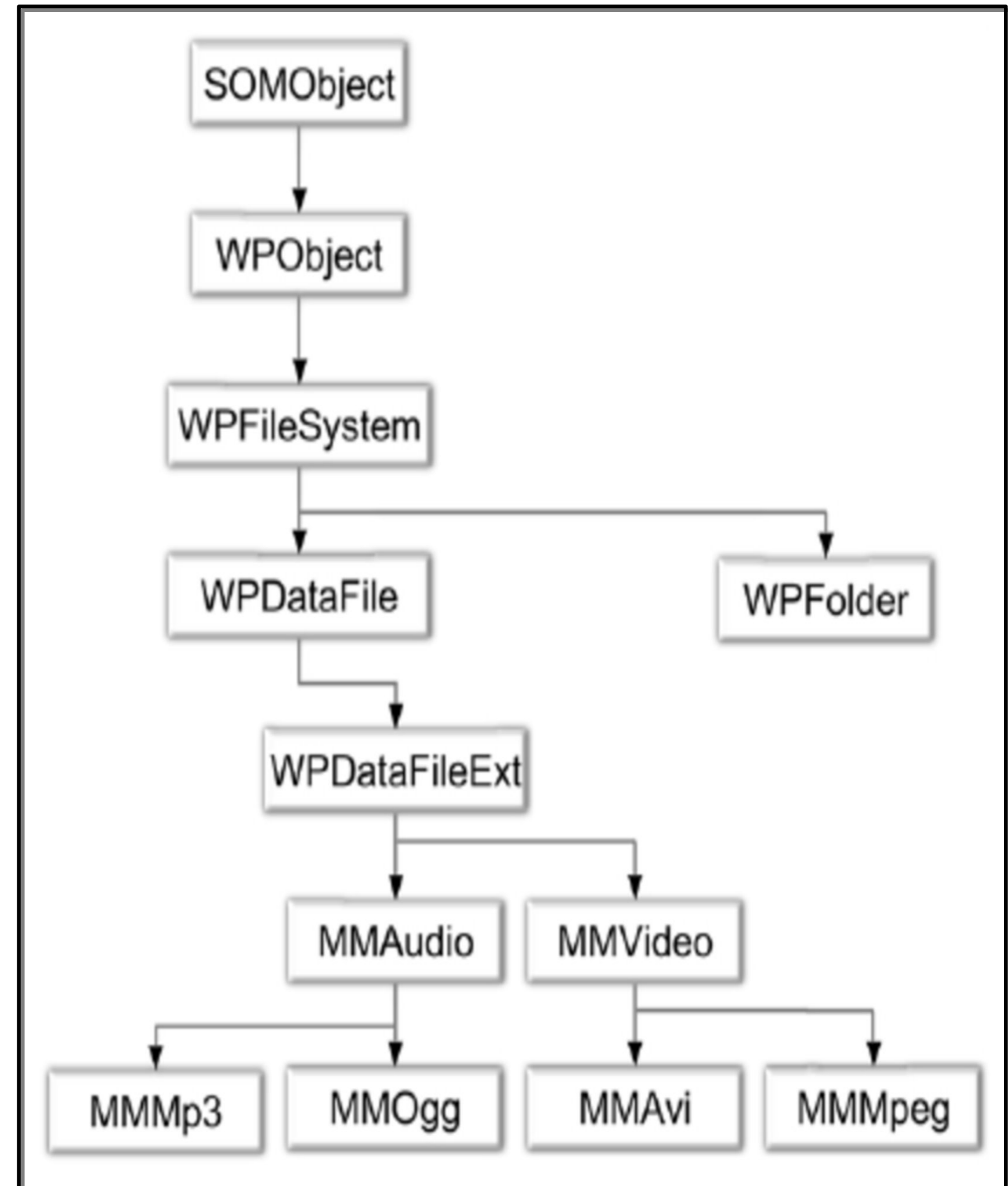
Objektorientierung am Beispiel: Die WPDataFileExt-Klasse ersetzt WPDataFile als Basisklasse für MMAudio und MMVideo.
